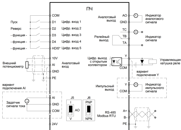
Рисунок 6 – Подключение управляющих клемм NC1 для моделей до 30 кВт
