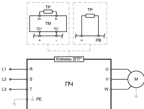
Рисунок 5 – Схема силовых подключений для моделей NCI-GY/PY-4B от 37 кВт
