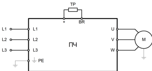
Рисунок 4 – Схема силовых подключений для моделей NCI-GY/PY-4B до 30 кВт
