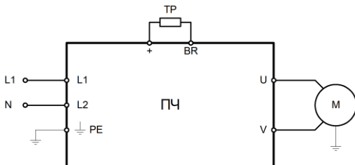
Рисунок 2 – Схема силовых подключений для моделей NCI-GY/PY-1B
