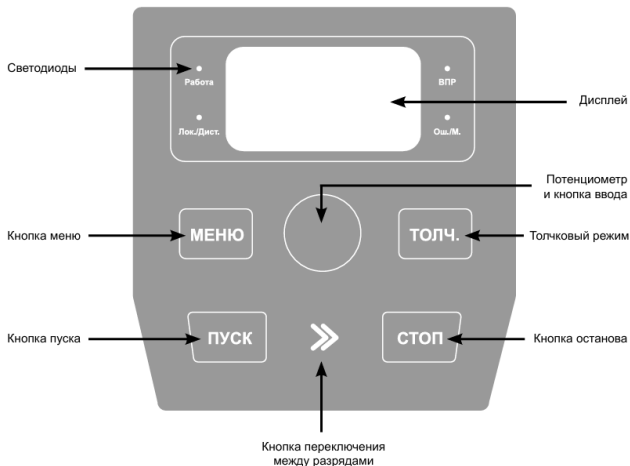
Рисунок 8 – Описание встроенной панели управления
