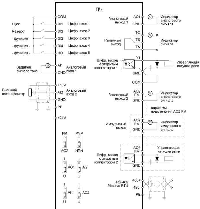
Рисунок 7 – Подключение управляющих клемм ПЧ для моделей от 37 кВт
