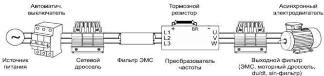
Рисунок 1 – Дополнительное оборудование
